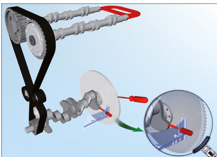
Figur 1: Registerremdrev med låseplate til kamaksel (rød) på plass, innstillingspinne til kamaksel (rød) og låseverktøy til svinghjul (rød)
