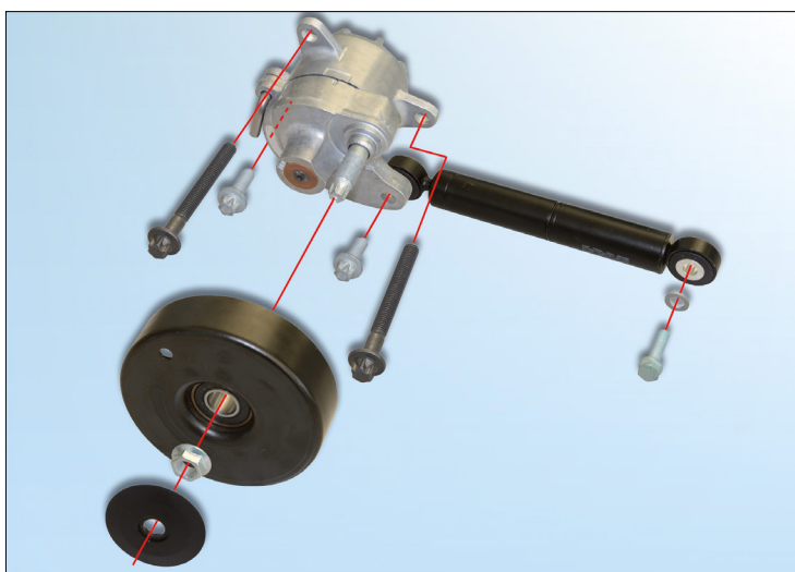
Fig. 1: 533 0116 10 – Set de reparații INA pentru ansamblul de antrenare inclusiv șuruburi de fixare
