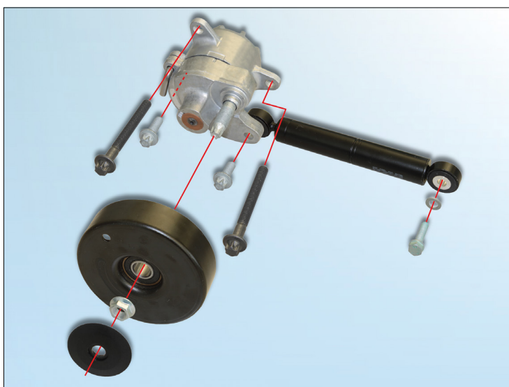
Снимка 1: 533 0116 10 – ремонтен комплект на INA за задвижвания на спомагателни възли, включително и фиксиращи болтове
