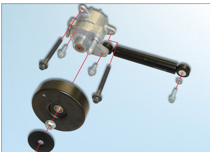
Obrázek 1: 533 0116 10 – opravářenská sada INA pro pohon agregátů včetně upevňovacích šroubů
