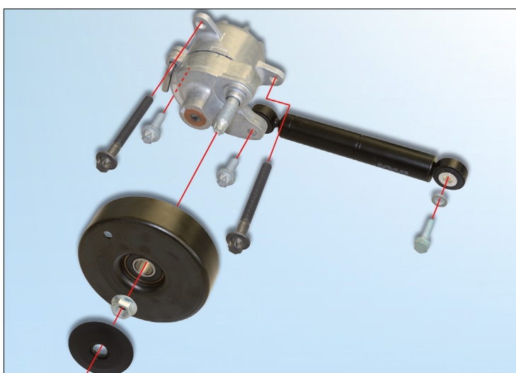
Figur 1: 533 0116 10 – INA reparationssæt til aggregatdrift inkl. fastgøringsskruer
