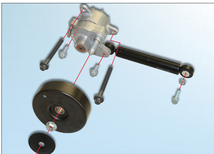
Εικόνα 1: 533 0116 10 – σετ επισκευής INA για το σύστημα κίνησης συμπεριλαμβανομένων και των κοχλιών στερέωσης
