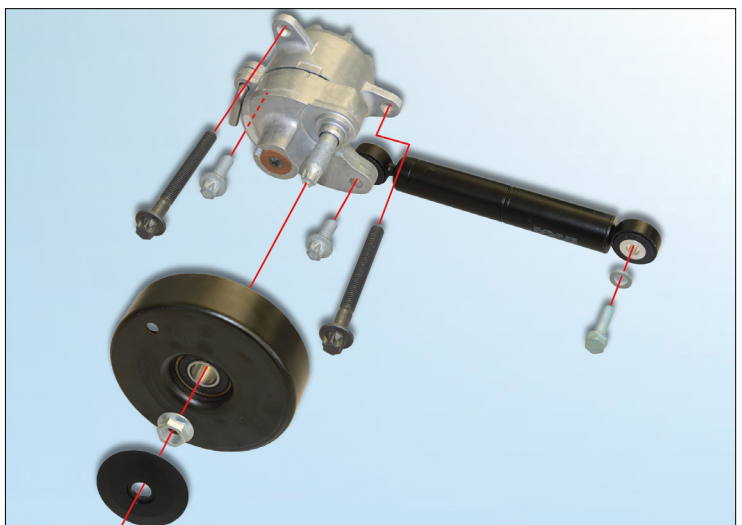
Kuva 1: 533 0116 10 – apulaitekäyttöjen INA-korjaussarja kiinnitysruuveineen
