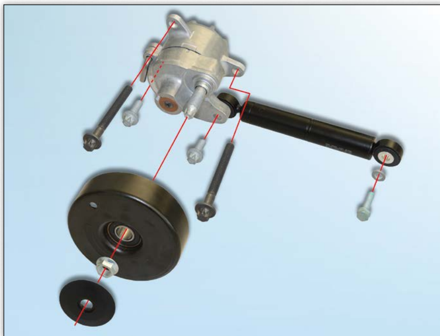
1. ábra: 533 0116 10 – INA javítókészlet a segédberendezések hajtásához a rögzítőcsavarokkal együtt
