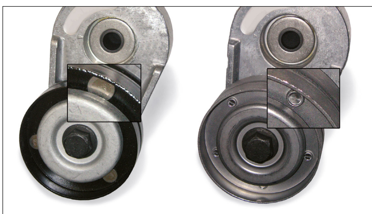
Figur 1: Detaljeret oversigt over skiverne i det tidligere design (venstre) og det nye design (højre)
