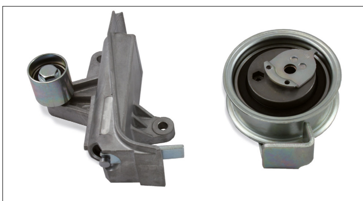
Figur 1: Vibrationsdæmper 533 0028 20 (venstre), strammer 531 0531 20 (højre)
