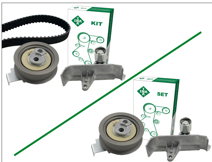
Kuva 2: Nykyinen malli, vasemmalla pidikkeellä varustettu ohjairulla 532 0601 10, oikealla kiristin 531 0840 10
