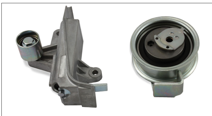
Kuva 1: Korvaantava malli, vasemmalla värähtelynvaimennin 533 0028 20, oikealla kiristin 531 0531 20
