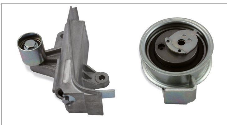
1. ábra: Balra az 533 0028 20 cikkszámú rezgéscsillapító, jobbra az 531 0531 20 cikkszámú feszítőgörgő
