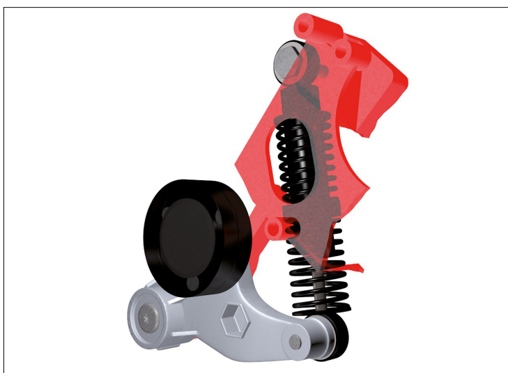
Fig. 1: Întregul ansamblu de tensionare
