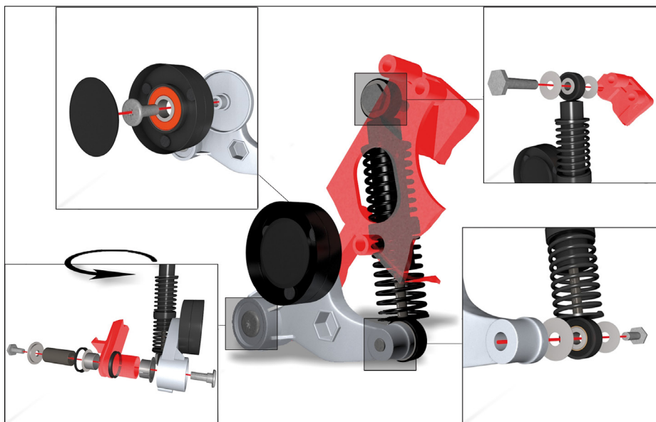
Obrázek 2: Přehled upevňovacích dílů
