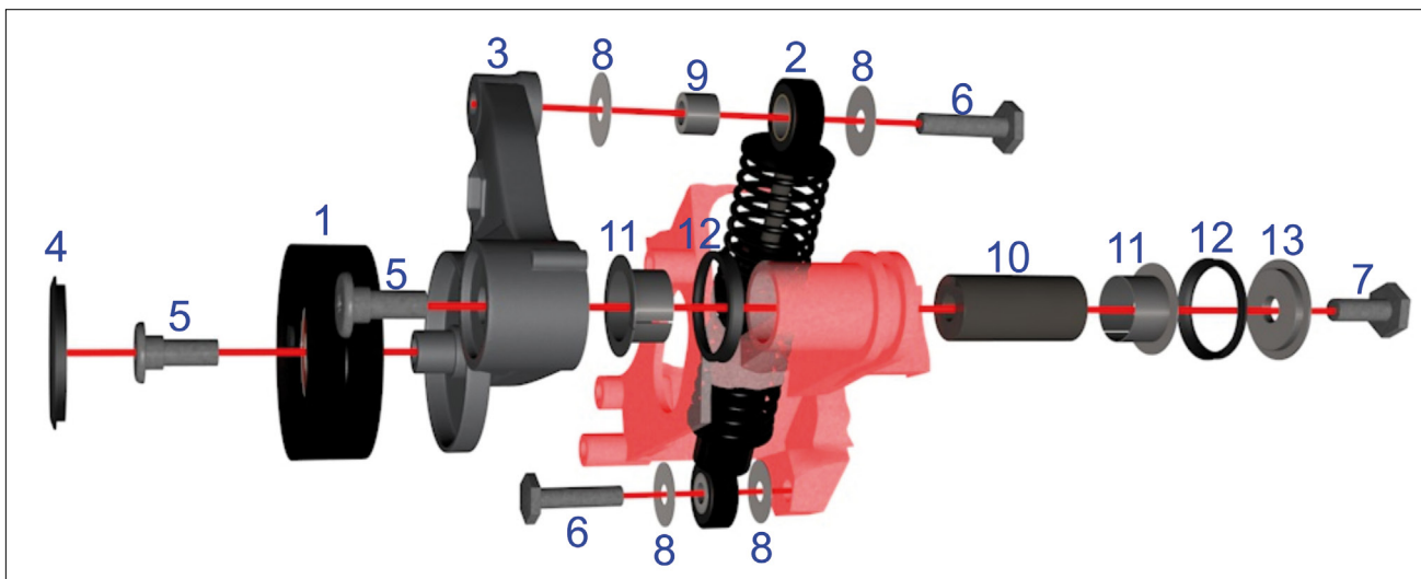
Obrázek 3: 533 0118 10 – INA-opravářská sada pro napínací jednotku
