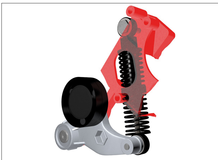
Obrázek 1: Kompletní napínací jednotka
