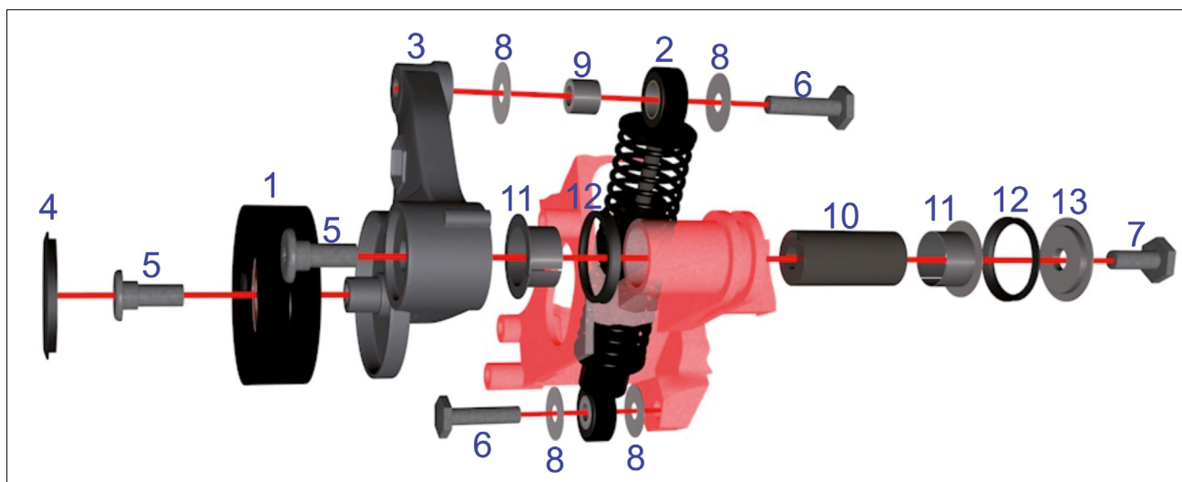
Figur 3: 533 0118 10 — INA reparationsset til strammeenhed
