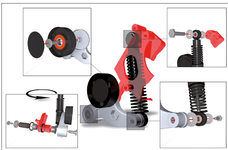
Figur 2: Oversigt over fastgørelsesdele
