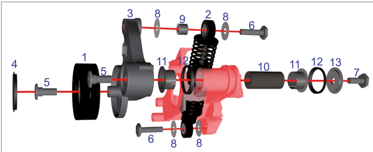
Kuva 3: 533 0118 10 – kiristinyksikön INA-korjaussarja
