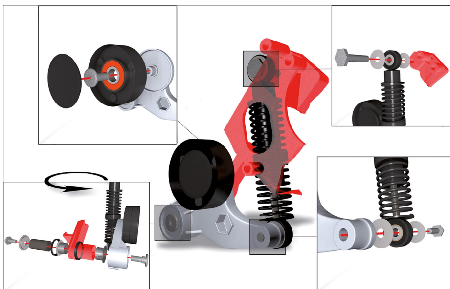
2. ábra: A rögzítő alkatrészek áttekintése
