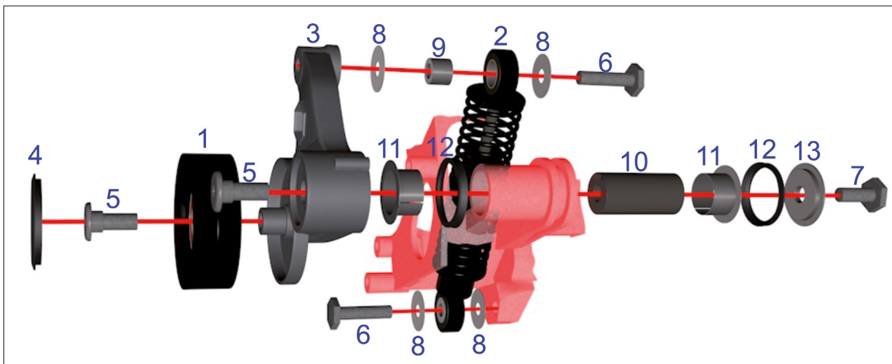
3. ábra: 533 0118 10 – INA javítókészlet a feszítőegységhez
