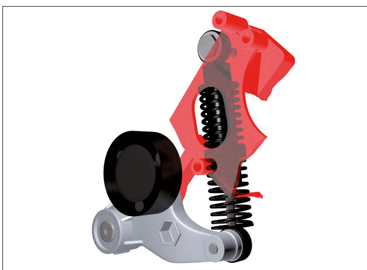
1. ábra: Komplett feszítőegység
