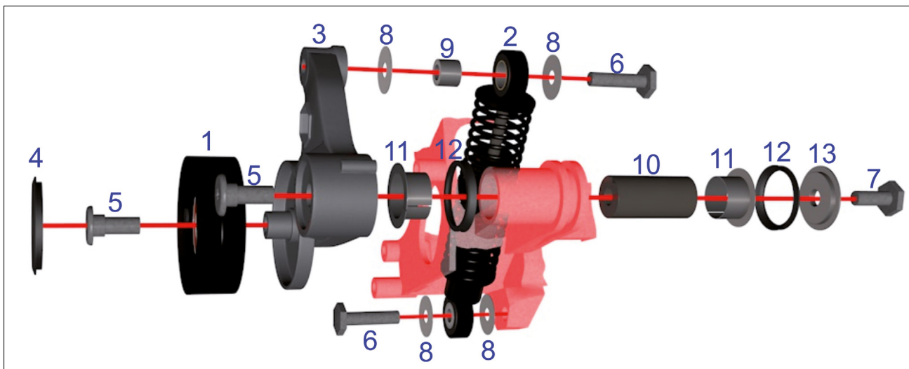
Bild 3: 533 0118 10 - INA reparasjonssats till remspännarenheter
