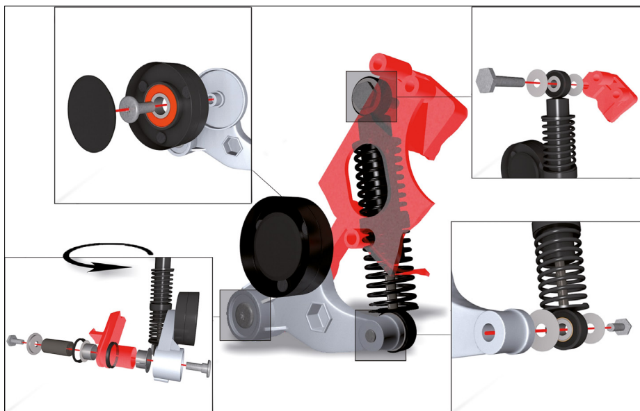
Bild 2: Översikt över fastsättningsdetaljer
