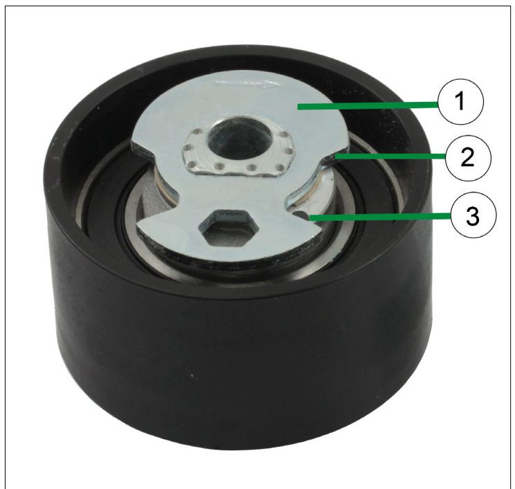
Kuva 1: 531 0504 10 – puoliautomaattinen kiristinpyörä
