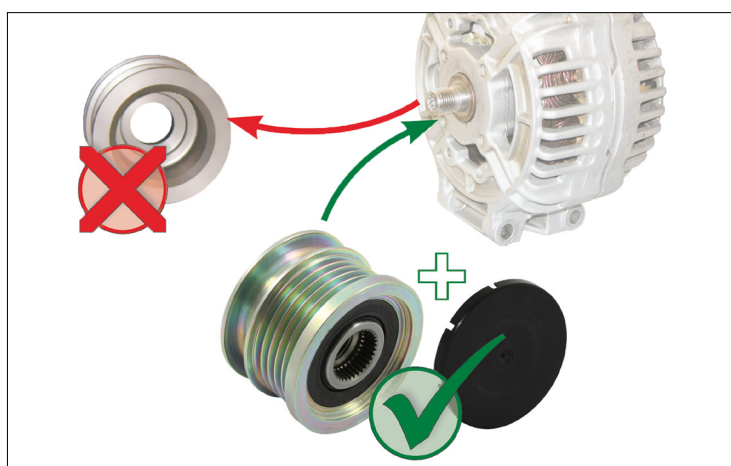
Obrázek 1: Výměna pevné řemenice za alternátorovou volnoběžku
