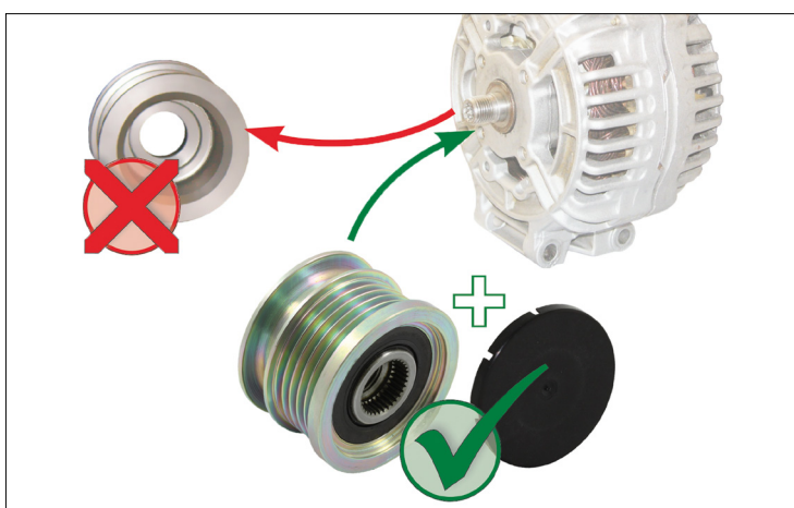
Figur 1: Udskiftning af en stiv remskive på en friløbsremskive
