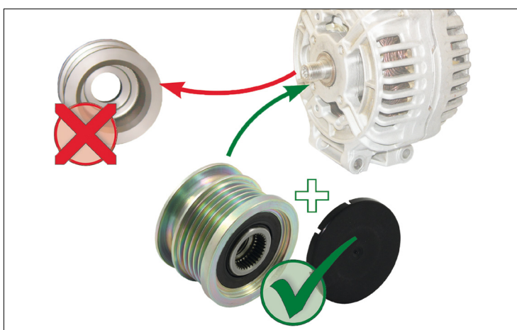
Εικόνα 1: Αλλάζοντας μια συμπαγή τροχαλία σε μία τροχαλία με κασάνια
