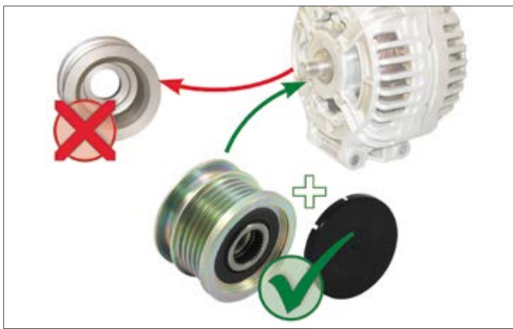
Рисунок 1: Замена цельного шкива на шкив генератора с обгонной муфтой
