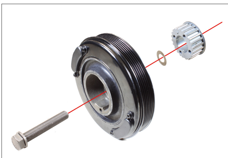
Figur 1: krumtapakselvibrationsdæmper med krumtapakselcentralbolt og diamantspændeskive
