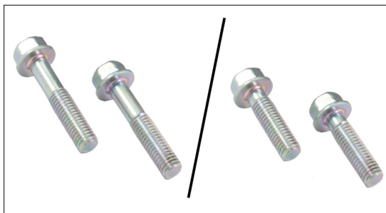
Fig. 4: Stânga, vechile şuruburi M8x40 mm. Dreapta, noile şuruburi M8x30 mm.
