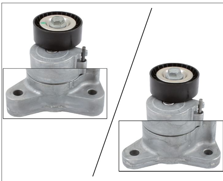
Obrázek 3: Vlevo, staré provedení s širšími upevňovacími body. Vpravo, nové provedení s užšími upevňovacími body.
