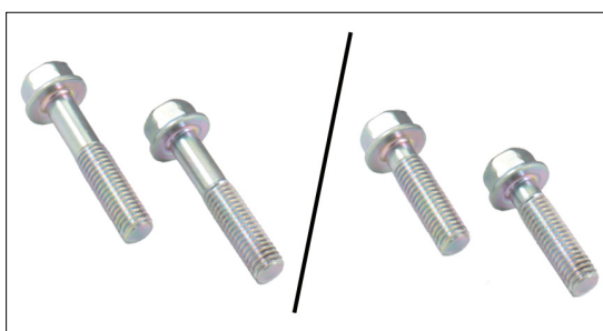
Figur 4: Venstre, gamle M8x40 mm bolte. Højre, nye M8x30 mm bolte.
