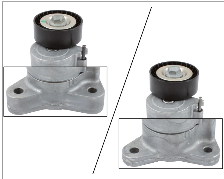
Εικόνα 3: Αριστερά, παλιά έκδοση με πλατιά σημεία στερέωσης. Δεξιά, νέα έκδοση με στενά σημεία στερέωσης
