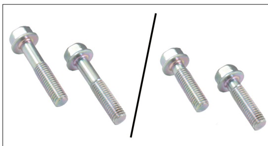
Bild 4: Till vänster, tidigare skruvar M8x40 mm. Till höger, nya skruvar M8x30 mm.
