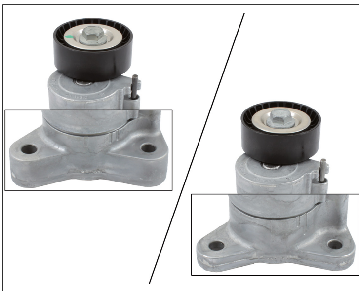
Bild 3: Till vänster, tidigare utförande med bredare fästpunkter. Till höger, nytt utförande med smalare fästpunkter.
