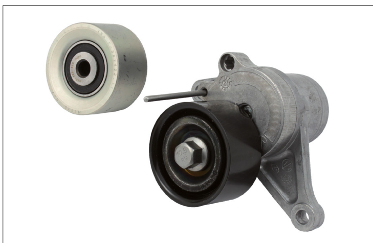
Fig. 1: Fulia întinzătorului și fulia deflectoare din metal
