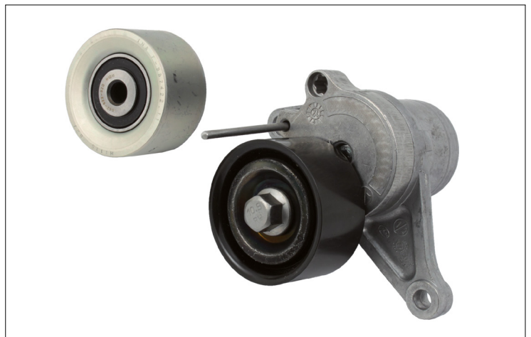
Εικόνα 1: Μεταλλική τροχαλία τάνυσης και τροχαλία εκτροπής
