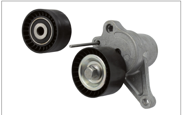
Εικόνα 2: Πλαστική τροχαλία τάνυσης και τροχαλία εκτροπής
