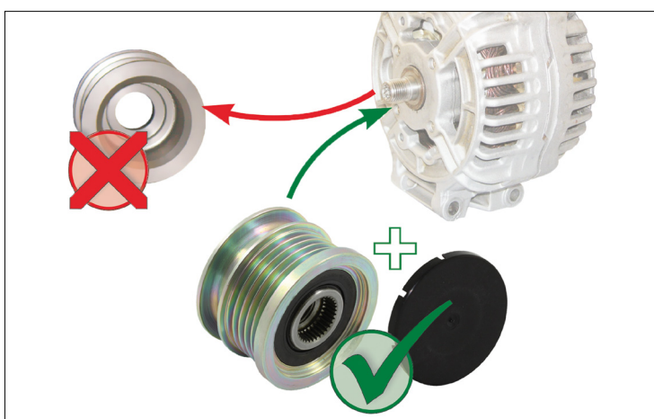
Εικόνα 1: Αντικαθιστώντας μια άκαμπτη τροχαλία ιμάντα με μια τροχαλία δυναμό με κασάνια
