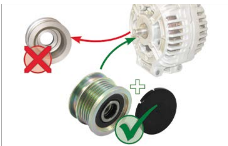
Рисунок 1: Замена жесткого шкива на шкив генератора с обгонной муфтой
