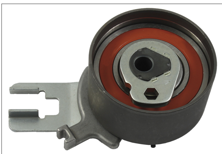
Fig. 1: 531 0859 10 — noua rolă de întindere
