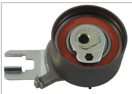
Снимка 2: 531 0515 10 — стария обтяжна ролка
