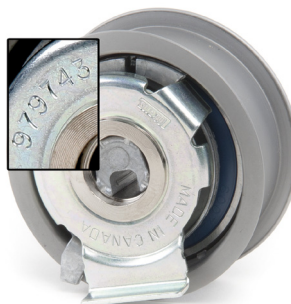
Фигура 1: 531 0777 10 – стария обтяжна ролка (979743)
