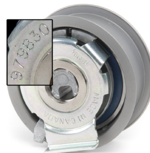
2. ábra: 531 0851 10 – új feszítőgörgő (979830)
