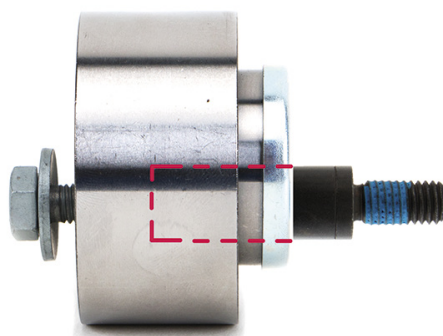
Снимка 4: Обтяжна ролка с втулка и монтаж болт в монтирано положение
