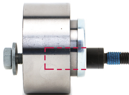
Kuva 4: INA-kiristinpyörä holkilla ja kiinnitysruuvilla asennusasennossa
