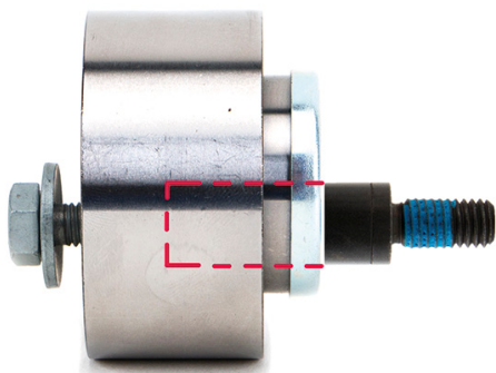
איור 4: גלגלת מותחן בעלת שריוול הברגה ובורג הידוק כאשר היא מותקנת למקומה
