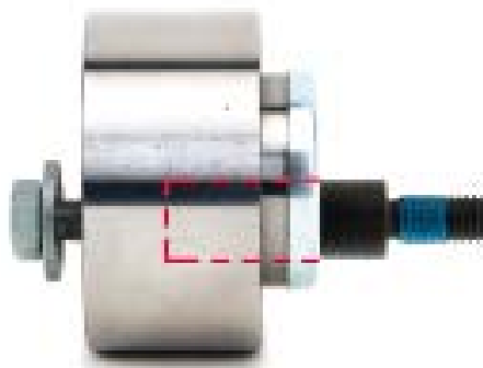
4. ábra: INA feszítőgörgő hüvelyes és rögzítőcsavarral a beszerelési helyzetben
