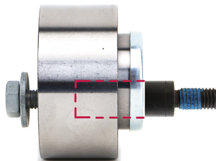
Bild 4: Spännrulle från INA med fäst- och hylsskruv i monteringsläge.
