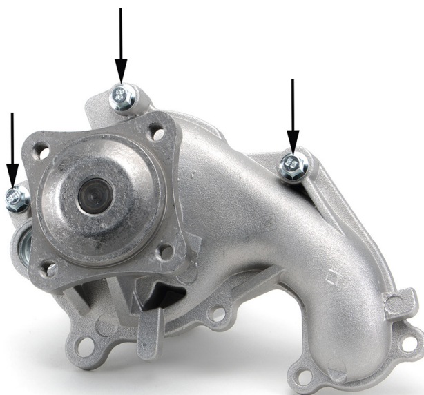
Снимка 2: Модифицирани точки за монтиране на помпата за охлаждаща течност
