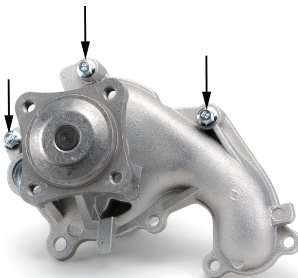
Obrázek 2: Modifikované upevňovací body čerpadla chladicí kapaliny
