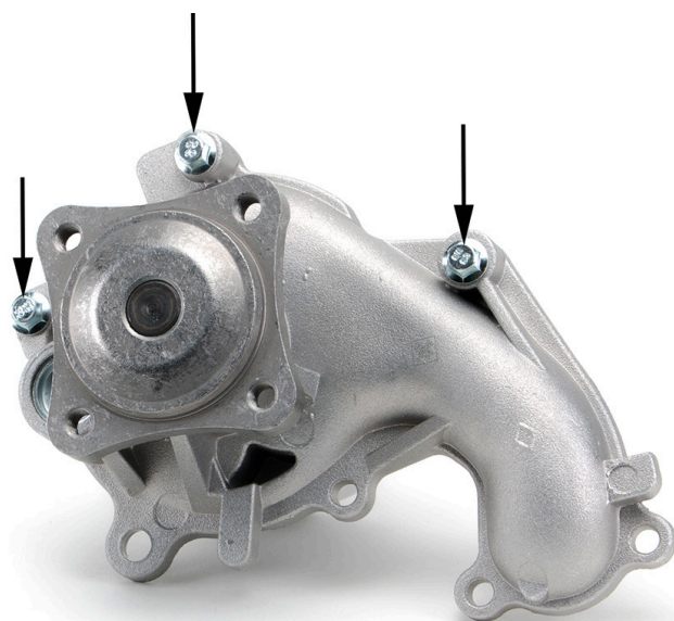
תמונה 2: נקודות בהן בוצע השיפור על משאבת המים
