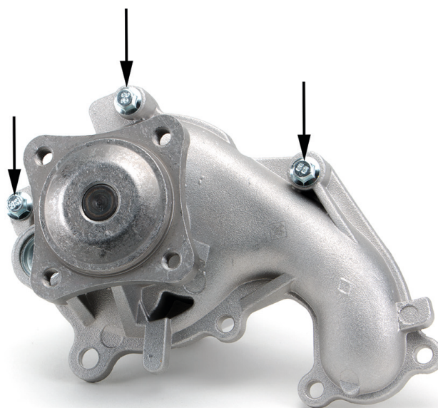
Figura 2: Punti di fissaggio modificati della pompa del liquido di raffreddamento
