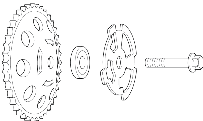
Снимка 2: Правилна монтажната последователност на всмукателния разпределителен вал при преобразуване от синтеровани към пресовани зъбни колела.
