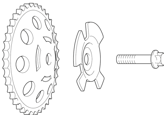
Kuva 4: Oikea asennusjärjestys imupuolen nokka-akselissa vaihdettaessa puristetusta teräksestä tehtyjä ketjupyöriä.
