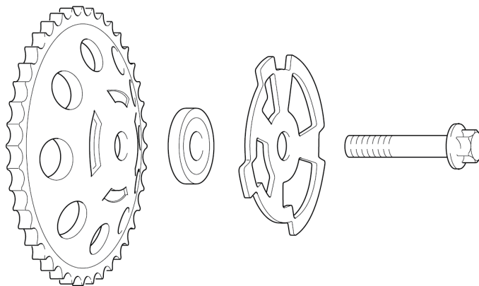
Kuva 2: Oikea asennusjärjestys imupuolen nokka-akselissa vaihdettaessa sintratusta materiaalista tehdyt ketjupyörät puristettuihin.
