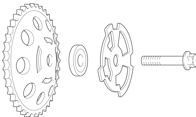
Fig. 2: Ordre de montage correct sur l'arbre à cames d'admission lorsque l'on remplace des pignons en métal fritté par des pignons en tôle d'acier découpée.
