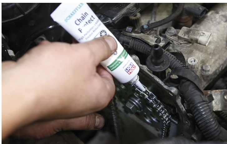
Bild 2: Tillsatsen Chain Protect från Schaeffler appliceras på alla komponenter i kedjedrivningen vid montering
